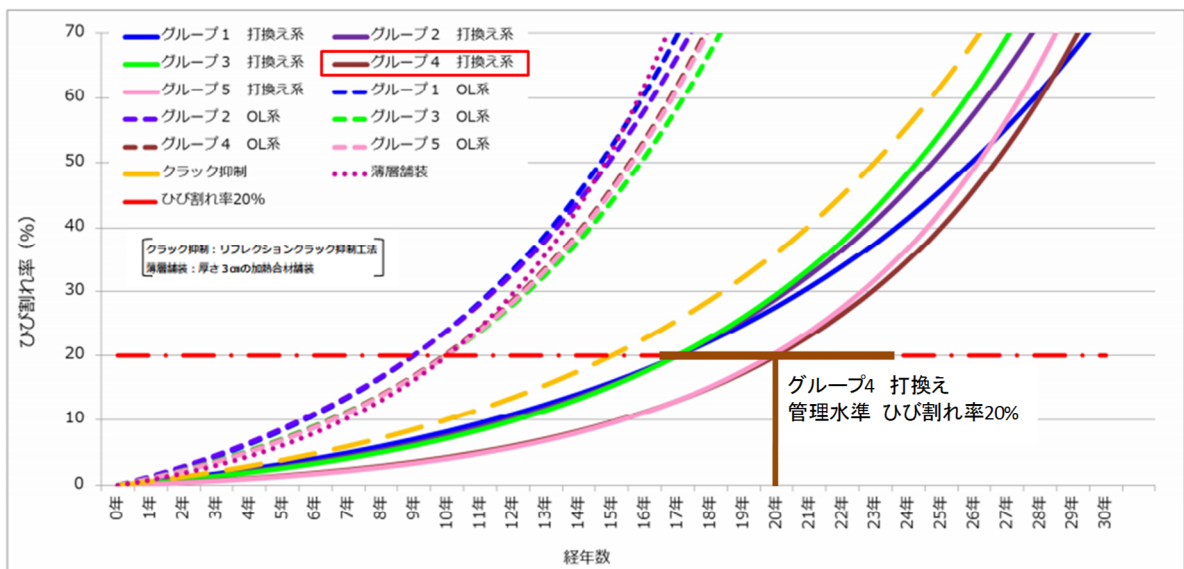
＜図 劣化予測式の例＞
