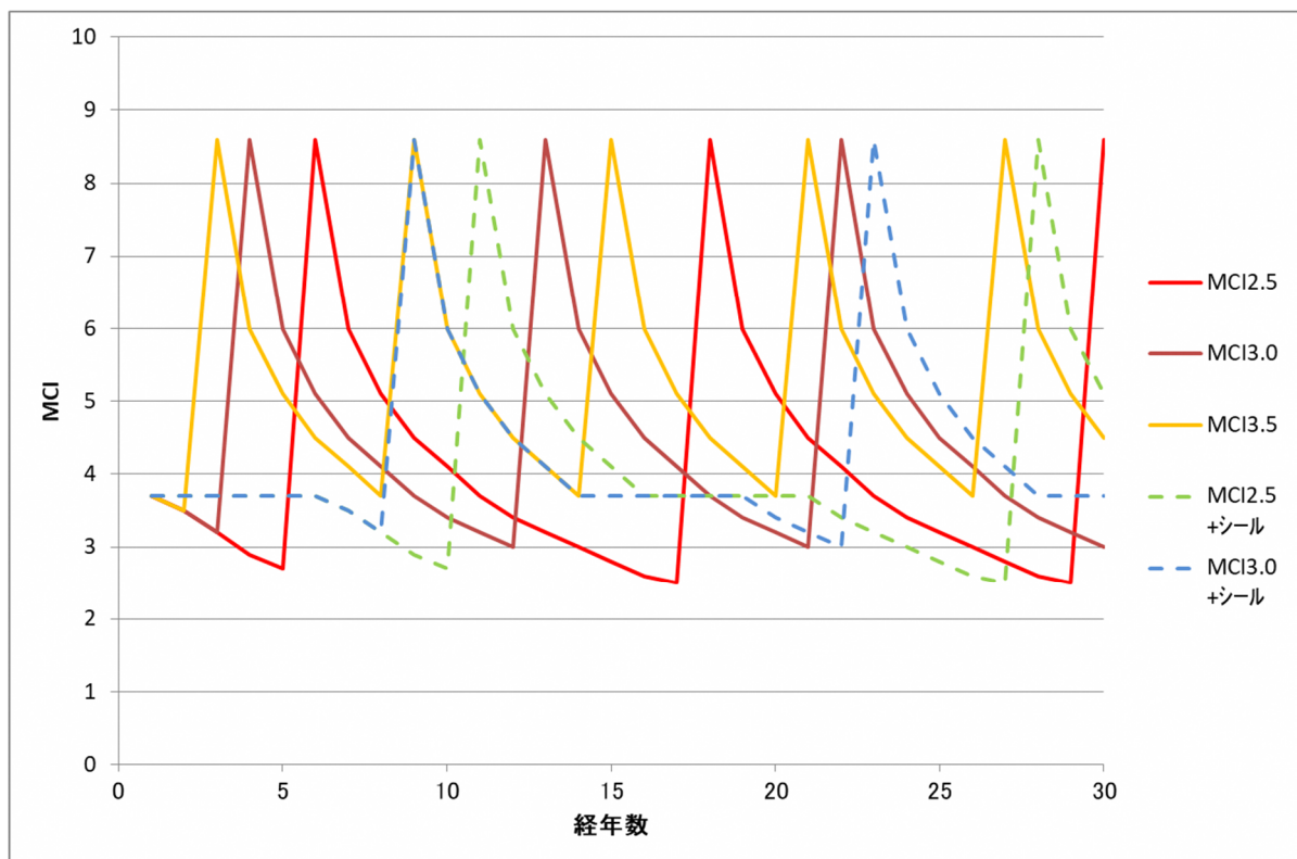
図- 3.2.1 修繕のタイミングおよびシール材注入による修繕回数比較
