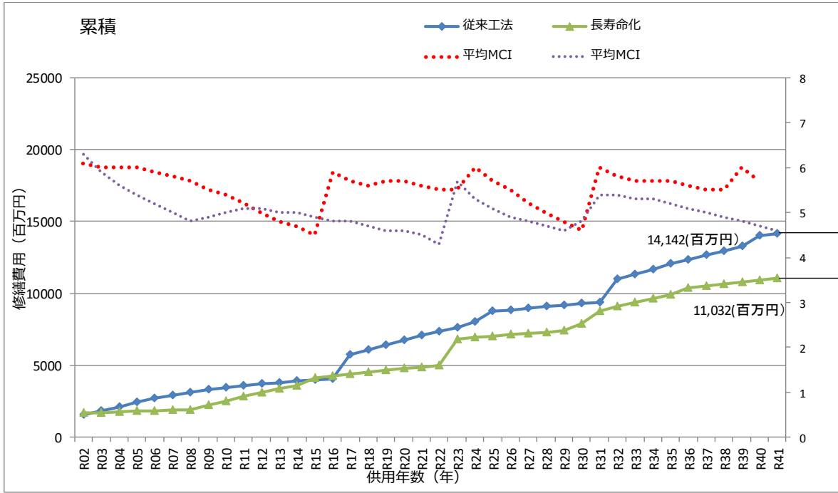
図-3.2.5 修繕費の試算結果
