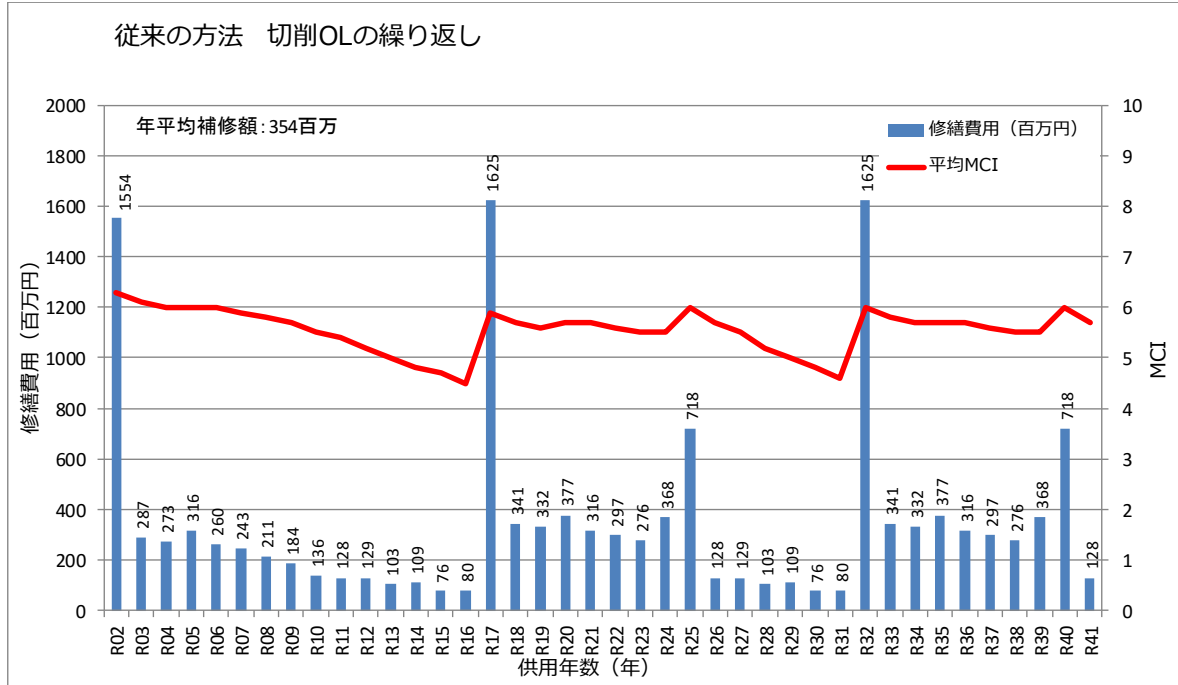
図-3.2.3 40年間の修繕費（従来の管理方法）
