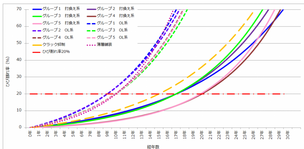
図-3.2.2 ひび割れ率の推移例(茨城県舗装維持修繕計画より抜粋)
