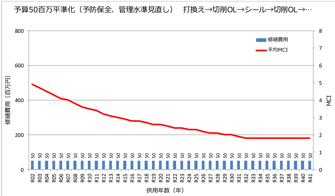
図-3.2.6 修繕費の試算結果（修繕費一定）
