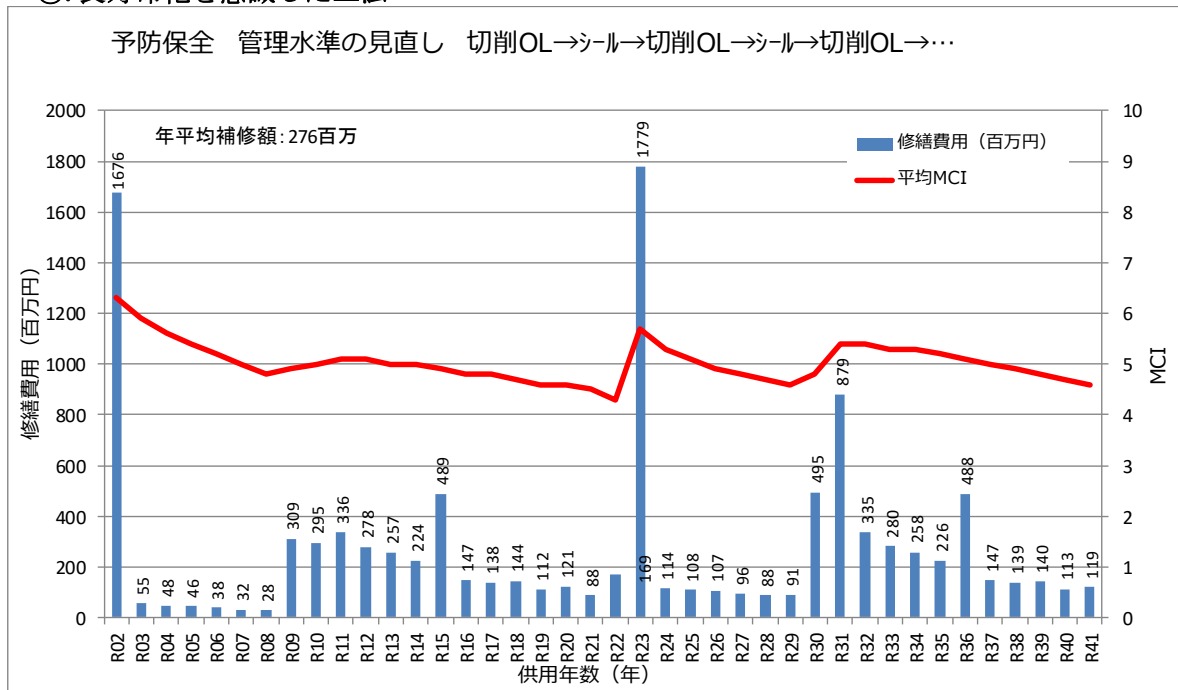
図- 3.2.4 40年間の修繕費（長寿命化を意識した管理方法）
